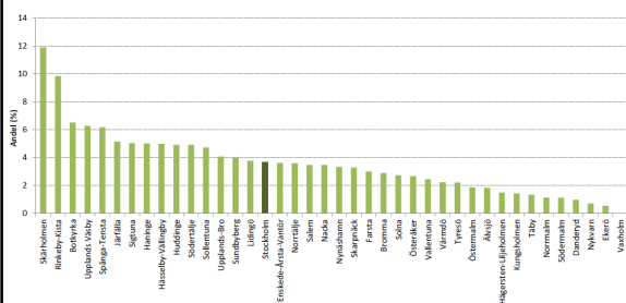
Tandhälsa mätt som andel (%) 3-åringar med kariesskadade tänder (deft) per kommun/stadsdel i Stockholms län 2016
